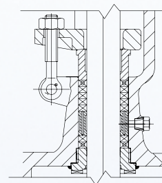
Sperrwasseranschluss
