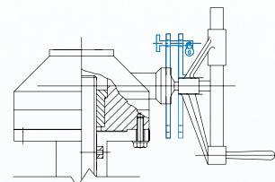
Tellerbefederte TA-Luft Stopfbuchspackung
