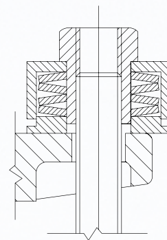
Tellerbefederte TA-Luft Stopfbuchspackung
